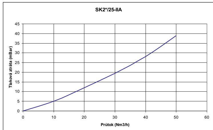
SK2P/25-IIA CL připojení CLAMP
